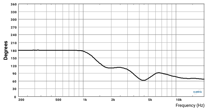
Horizontal Beamwidth
