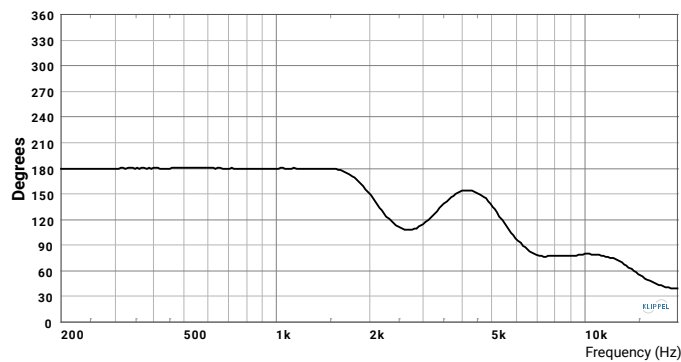
Horizontal Beamwidth
